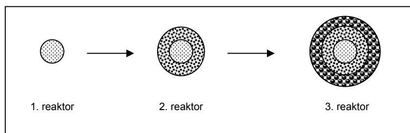
2. ábra A polimer részecskék szerkezetének változása a reaktorsorban
