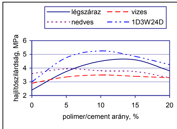
5. ábra A polimer (SBR latex)/cement arány hatása az EPS tartalmú betonok hajlítószilárdságára különböző érlelési körülmények (légszár, vizes, nedves és kombinált: 1D3W24D = 1 nap száraz+3 nap vizes+ 24 nap száraz) érlelés után
