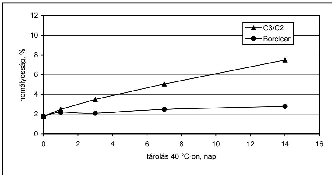
5. ábra Magas etiléntartalmú, 80 \mu m vastag C_3/C_2 és Borclear fólia homályosságának változása a 40 °C-on végzett tárolás időtartamának függvényében
